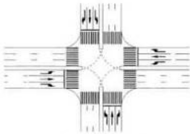
Marcaj de ghidare la intersecție
