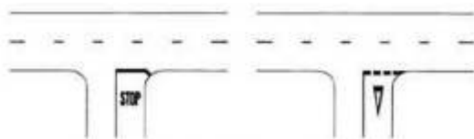
Marcaj de oprire și cedare a priorității
