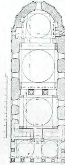
Fig. 190. — Plan
