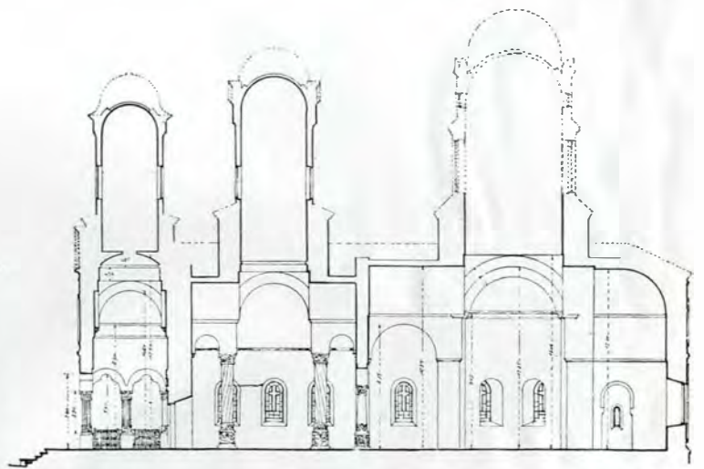
Fig. 300. — Coupe
