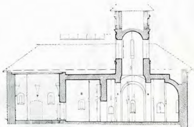
Fig. 76. — Coupe
