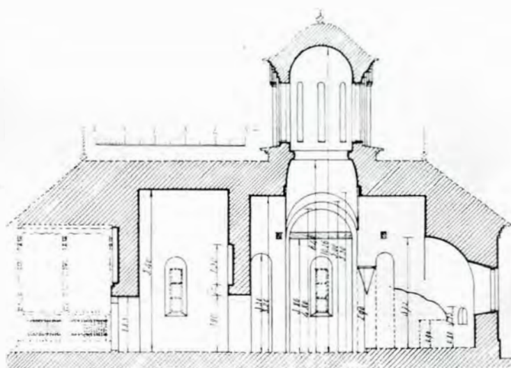
Fig. 73. — Coupe
