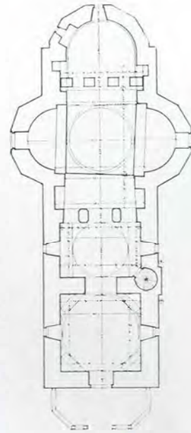
Fig. 217. — Plan
