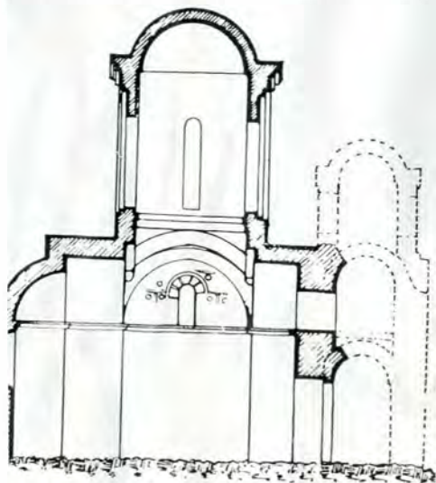
Fig. 39. — Coupe
