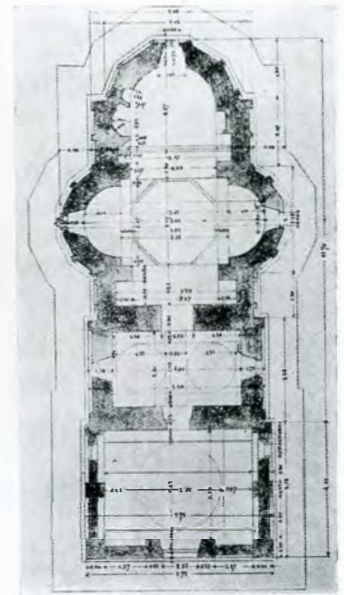
Fig. 162. — Plan
