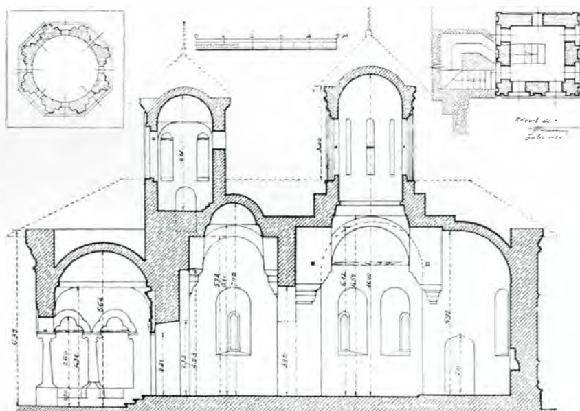
Fig. 225. — Coupe
