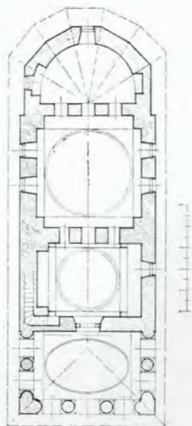
Fig. 285. — Plan
