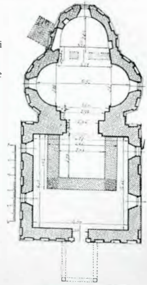
Fig. 132. — Plan
