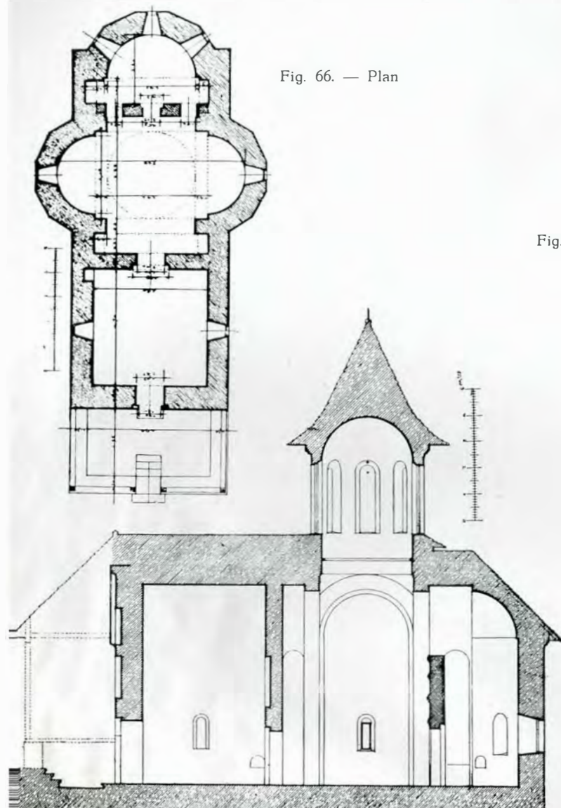
Fig. 67. — Coupe
