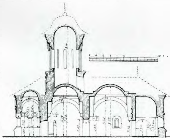
Fig. 330. — Coupe
