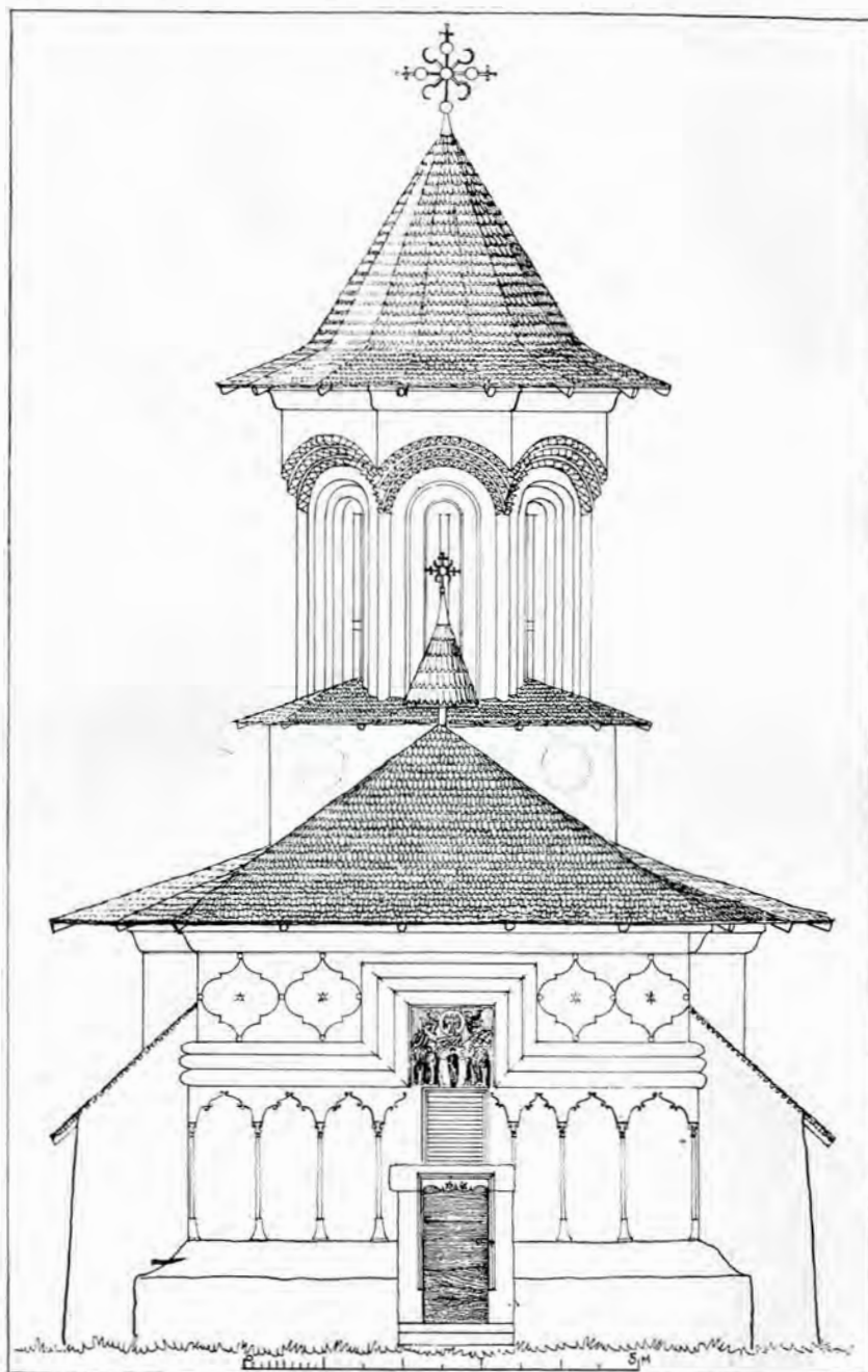
Fig. 5. — Biserica Schitului Mărculeşti-Flămânda. Faşada principală restituită după fotografii.
