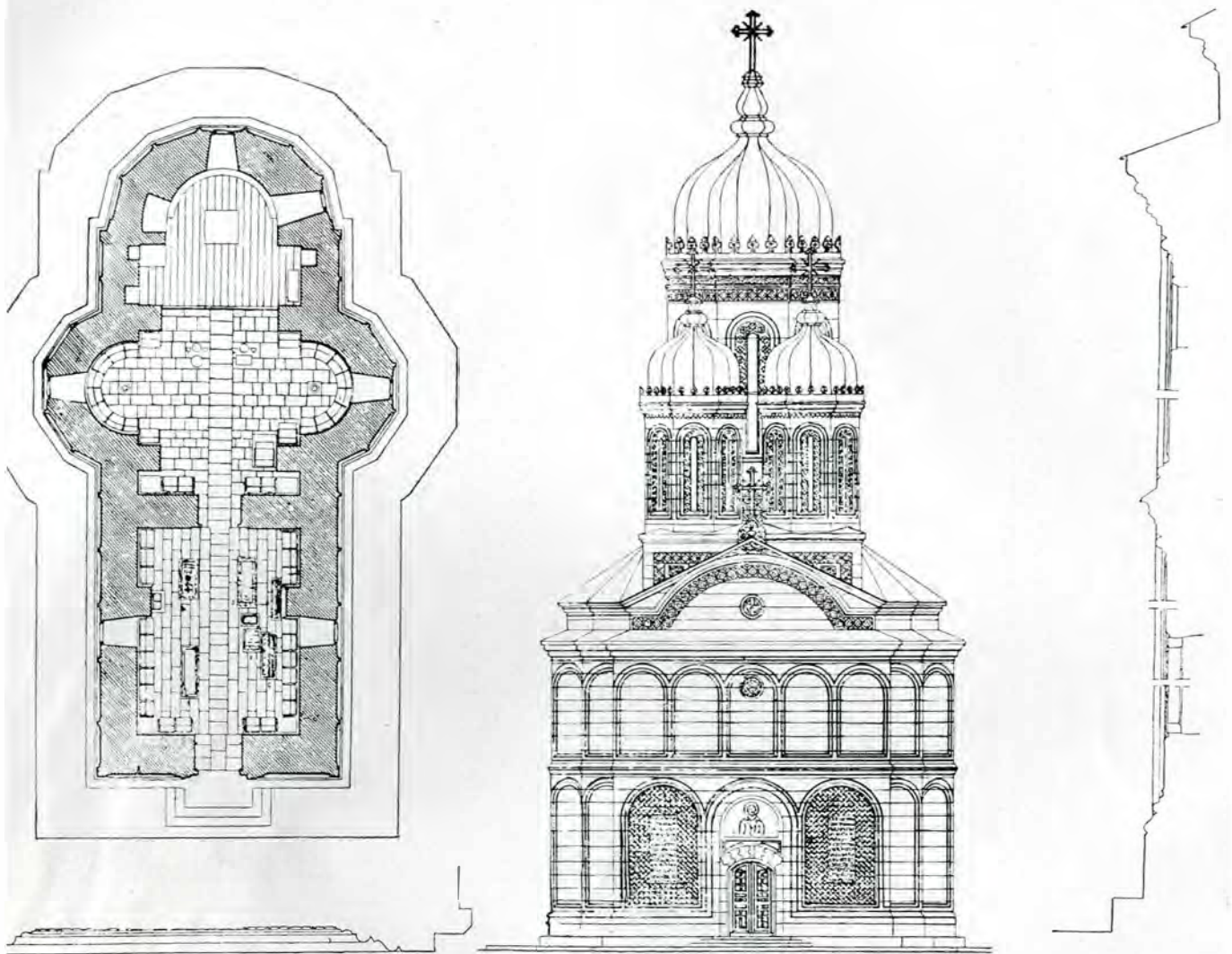
Fig. 78. — Plan
