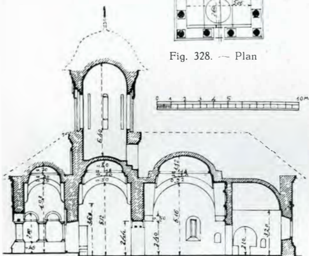
Fig. 331. — Coupe
