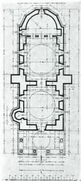
Fig. 279. — Plan
