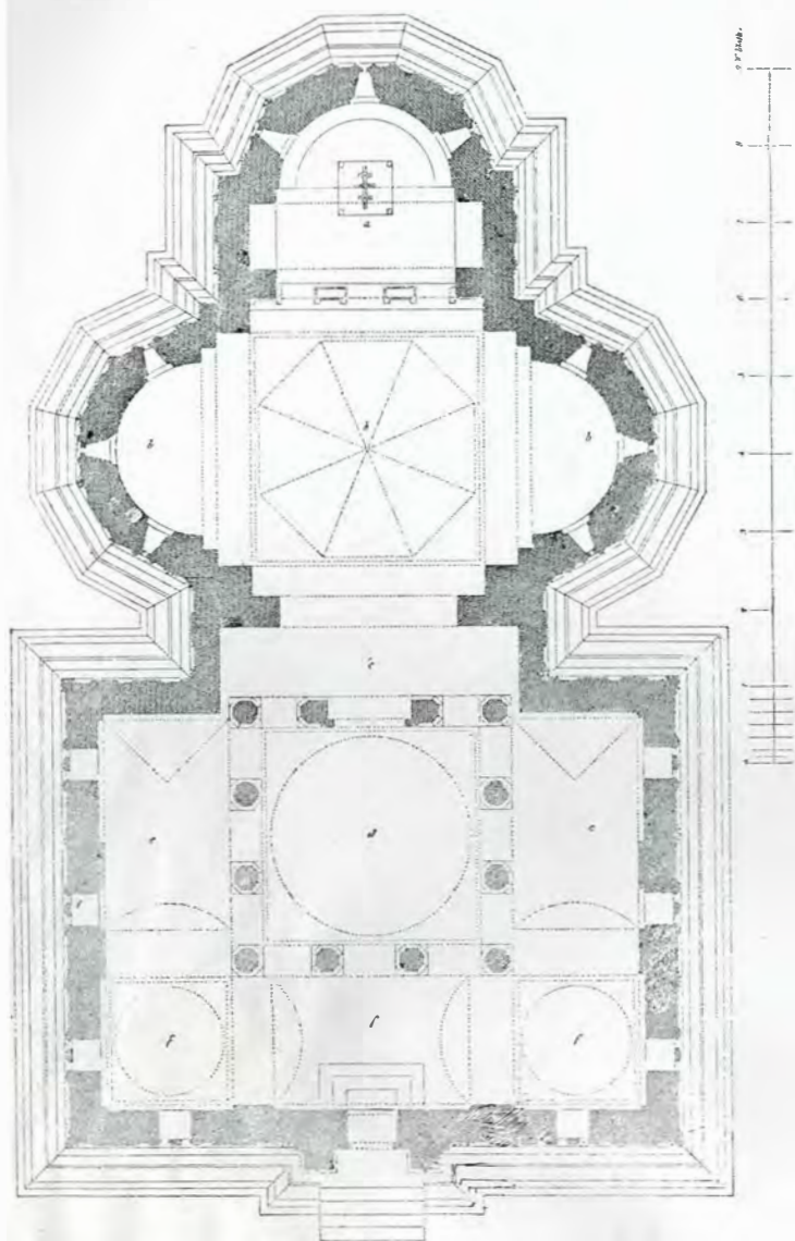
Fig. 88. — Plan
