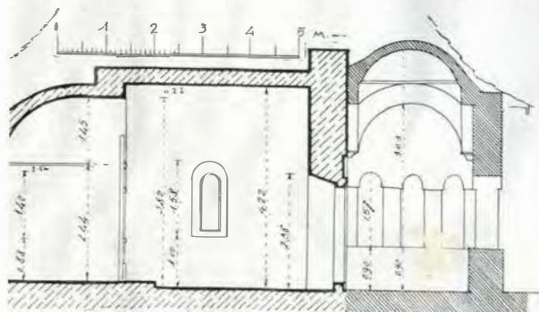
Fig. 101. — Coupe
