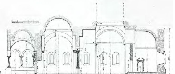
Fig. 199. — Coupe
