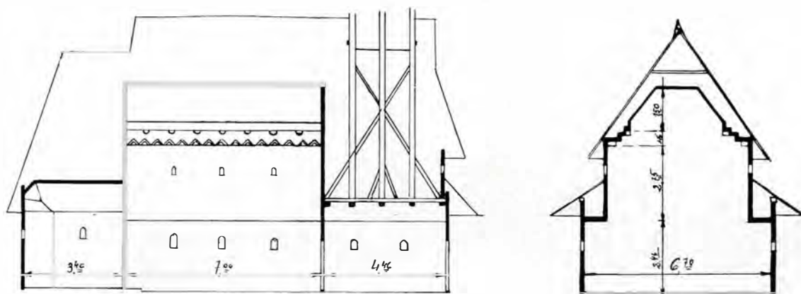
a. Biserica din Ieud. — Secțiuni la biserica din deal.
