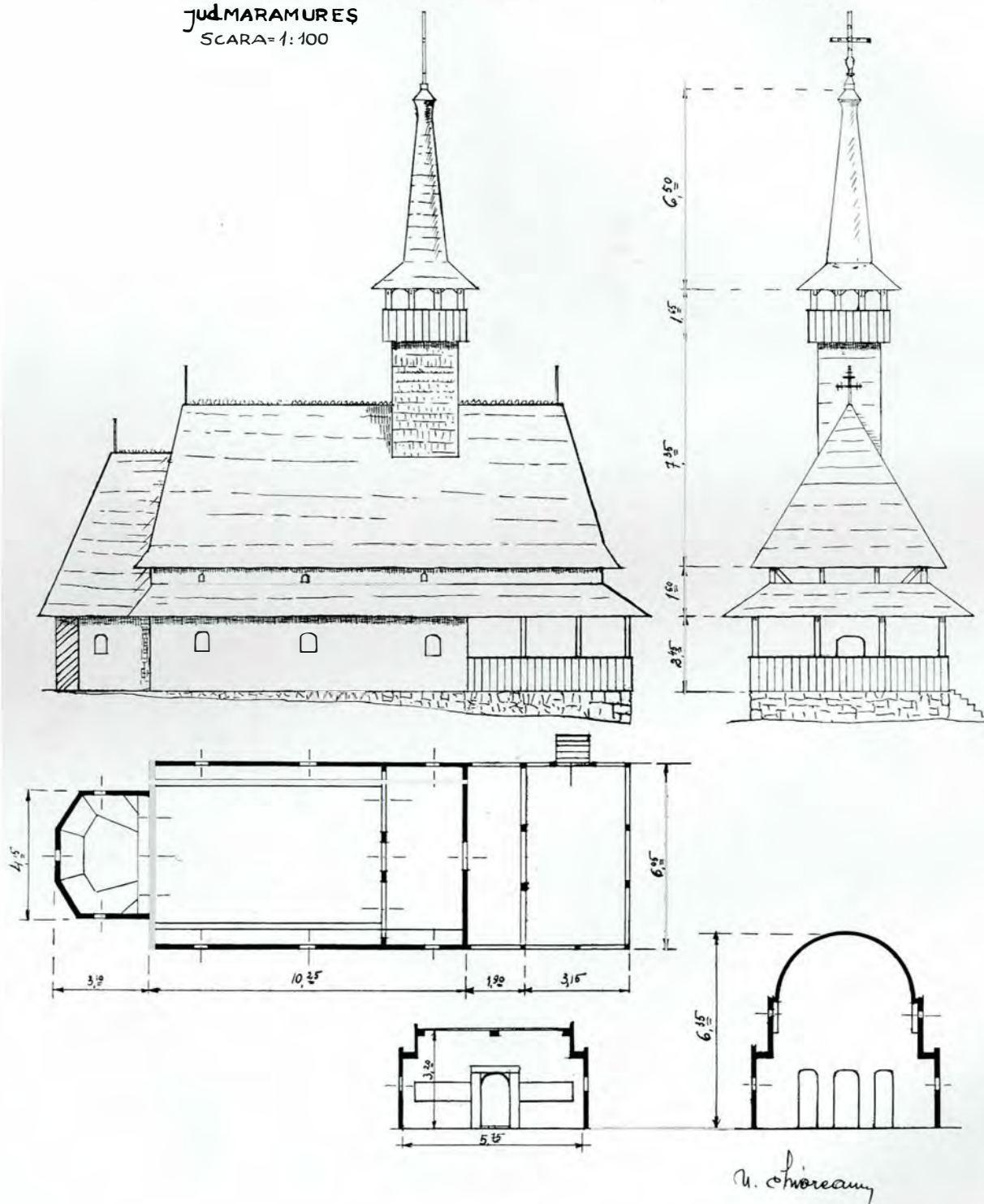
Biserica din Selistea-de-Sus. — Plan, secţiuni, vederi.
