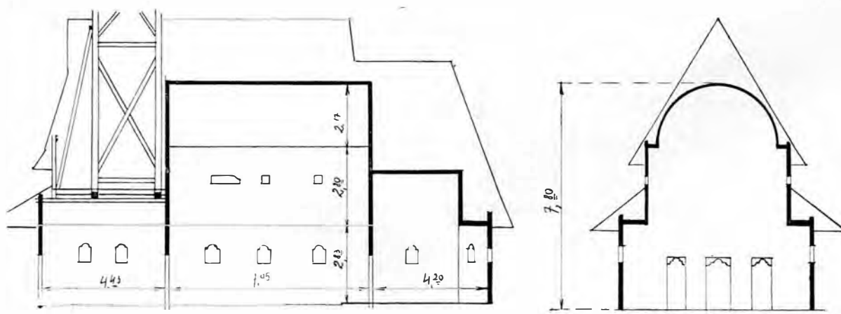
b. Biserica din Ieud. — Secțiuni la biserica din vale.
