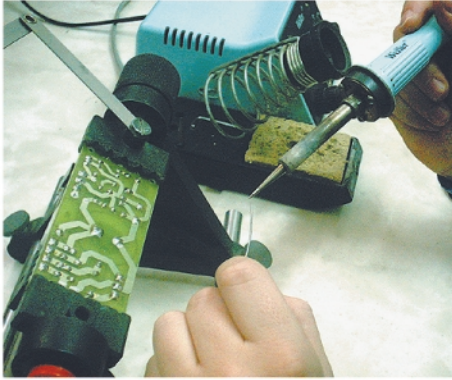
Fig. 1 Relevant pentru transferul de căldură
