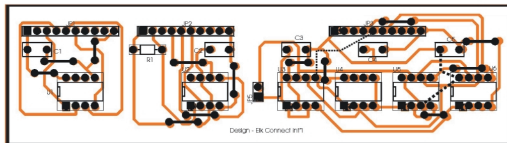
Fig. 6 Amplasarea componentelor pe cablajul adaptorului
