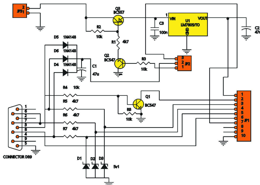
Fig. 1 Schema electrică a interfeței
