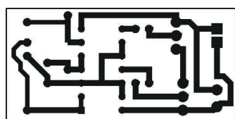
Fig. 2a Cablajul oscilatoru- lui
