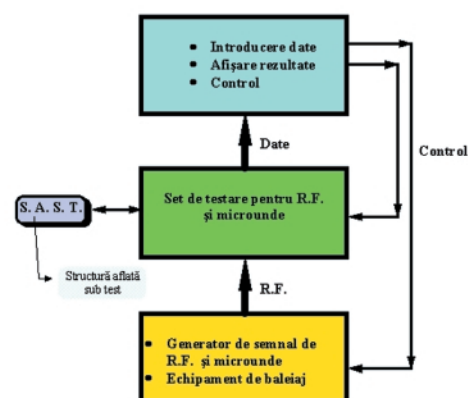
Fig. 7 Schemă bloc a unui analizor vectorial de rețea ("Vector Network Analyzer")
