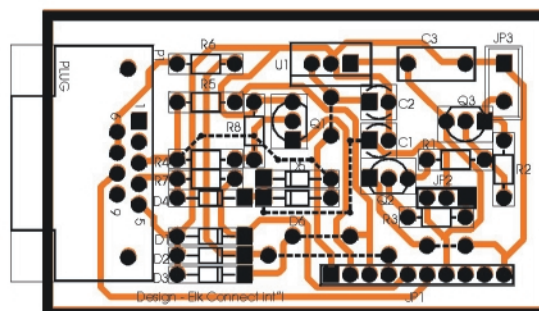
Fig. 4 Amplasarea componentelor la cablajul interfeței
