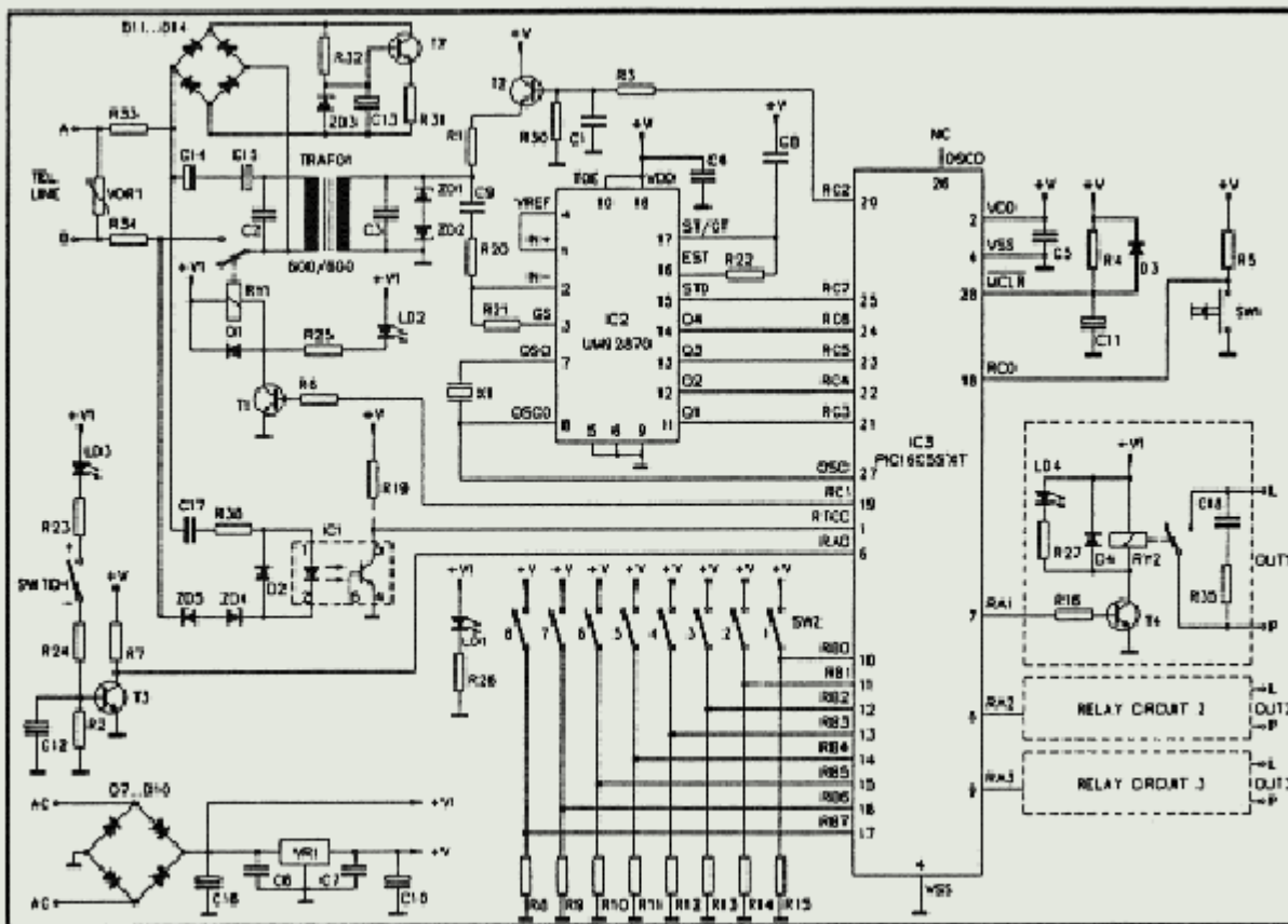
Fig. 1 Schema electrică de principiu
