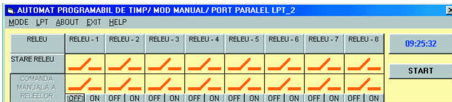
Fig. 3 Interfața grafică pentru modul de lucru manual
