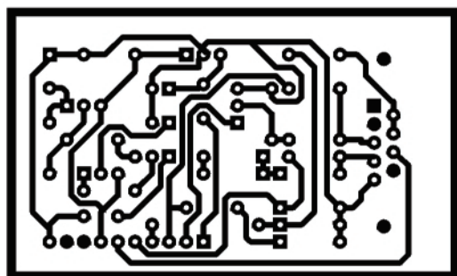
Fig. 3 Cablajul interfeței
