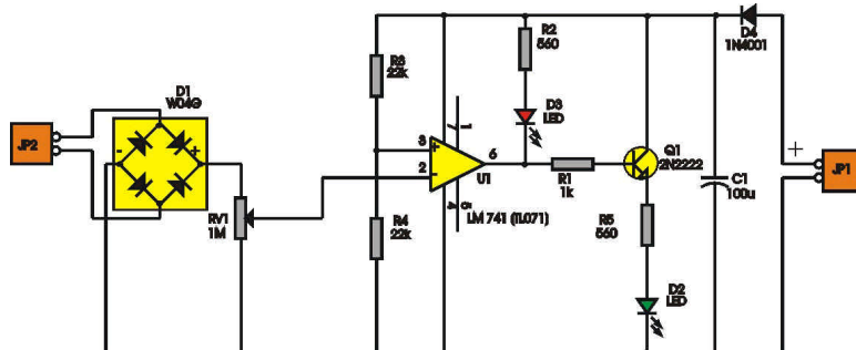
Fig. 1 Schema electrică
