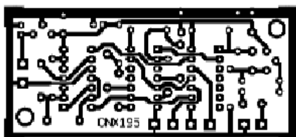
Fig. 3 Desenul cablajului imprimat
