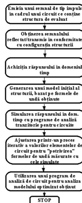
Fig. 10 Diagrama de desfășurare a procesului TDMT
