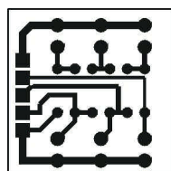
Fig. 3 a Cablajul multiplicatorului
