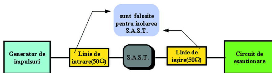
Fig. 9 Tehnică de calibrare folosind linii adaptate pentru izolarea S.A.S.T.
