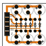
Fig. 2a Cablajul oscilatoru- lui
