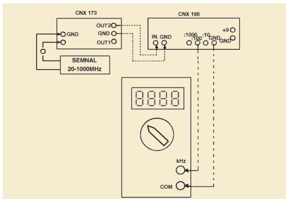
Fig. 1 Montaj de măsură pentru extindere la 1GHz
