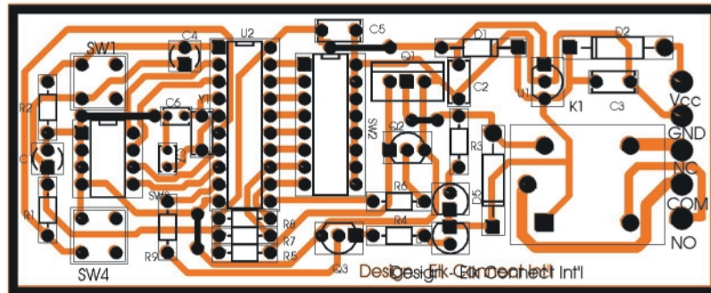
Fig. 5 Amplasarea componentelor
