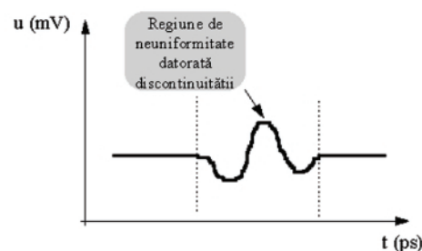
Fig. 6 Schiță a unei forme de undă modificate datorită existenței în structura de interconectare a unei discontinuități
