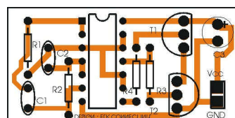
Fig. 2b Desenul de amplasare- al oscila- torului
