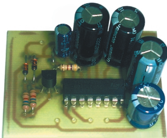
Fig. 5 a Cablaul imprimat al interfeței
