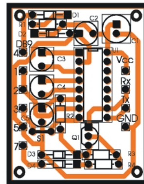
Fig. 5 b Desenul de amplasare a compo- nentelor
