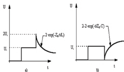
Fig. 12 Vizualizarea formelor de undă pe ecranul reflectometrului în cazul:
