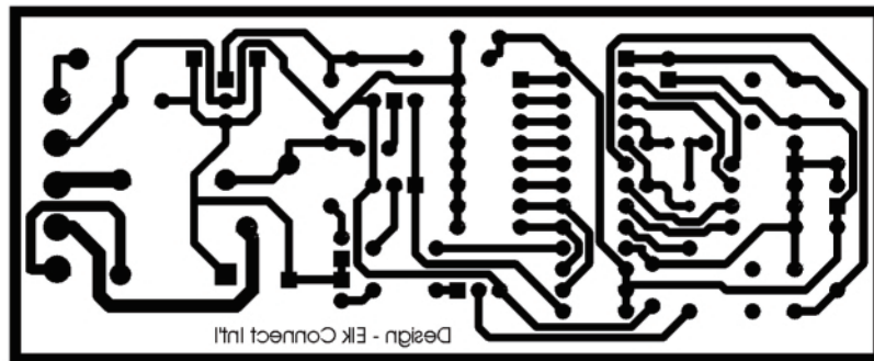
Fig. 4 Desenul cablajului imprimat
