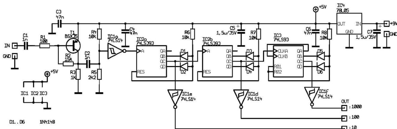
Fig. 2 Schema electrică
