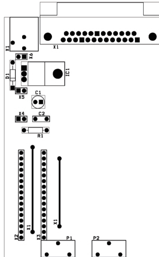
Fig. 3 Layer de inscripționare
