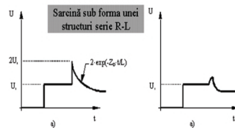
Fig. 13 Vizualizarea formelor de undă în cazul unei sarcini serie R-L:
