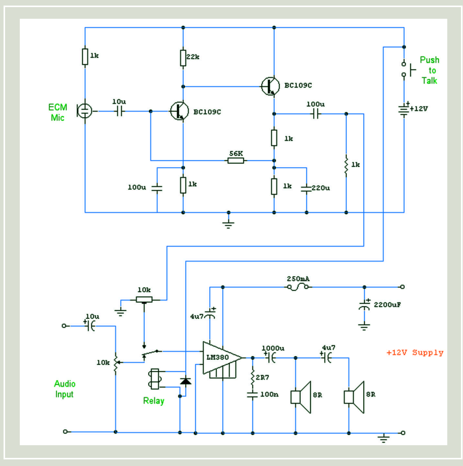
Fig. 1 Schema electrică
