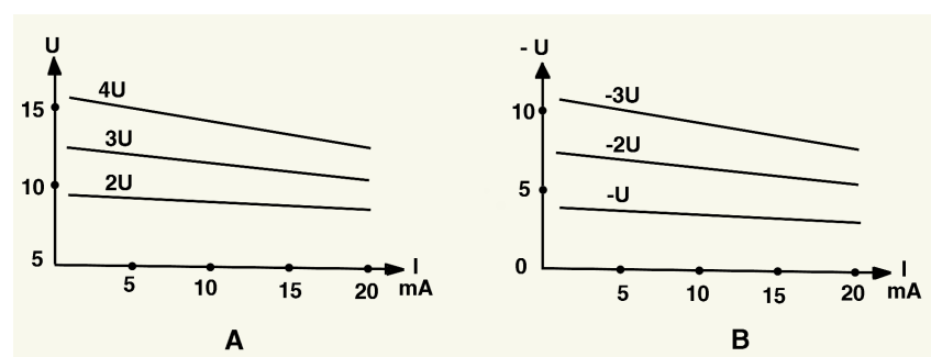
Fig. 4 Varoarea tensiunii funcție de curentul prin sarcină
