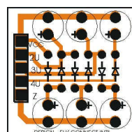
Fig. 3 b Desenul de amplasare pentru tensiuni pozitive
