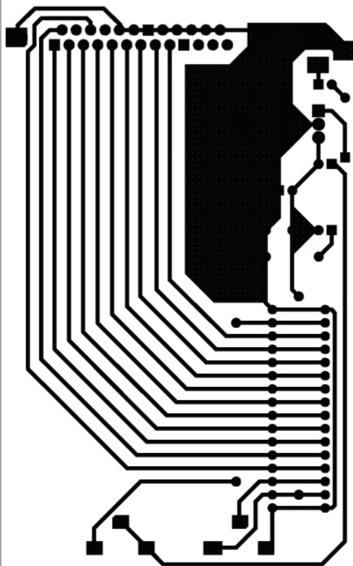
Fig. 2 Layer trasee
