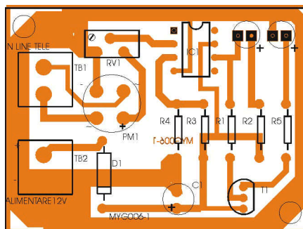
Fig. 3 Desenul de amplasare
