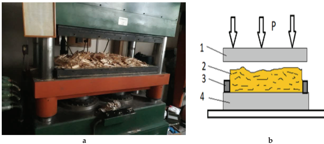
Figura 5. Presa hidraulică de presare a covorului (a) și rolul distanțierelor în timpul presării. Legendă: 1 - platan superior, 2 - covor de așchii, 3 - distanțiere, 4 - platan inferior.
