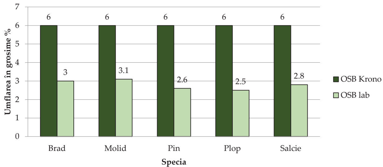
Figura 9. Comparație între umflarea plăcilor de laborator și cea specifică plăcilor obținute industrial. Legendă: OSB Krono - plăci preluate de pe linia de fabricație a fabricii, OSB lab - plăci obținute în condiții de laborator respectând tehnologia din fabrică (așchii, adeziv etc.)
