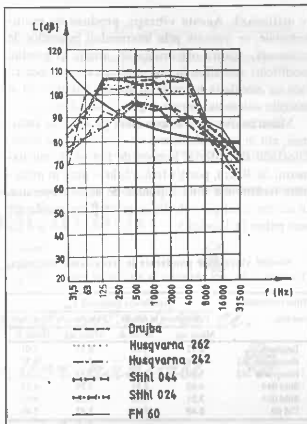
Fig. 2. Diagrama spectrală a zgomotelor produse de ferăstraiele mecanice „la secționarea arborilor”, în dB. (The spectral diagram of the noises produced by mechanical saws by the cross cutting of the trees” in dB).
