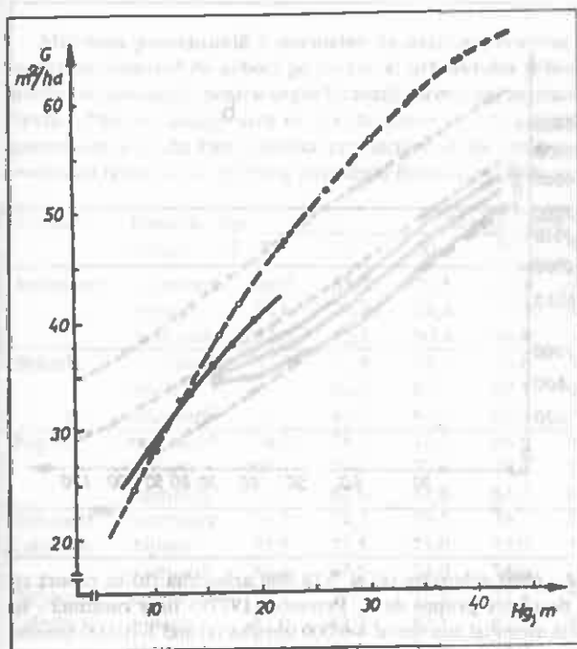
Fig. 1. Comparație între variația densității molidișurilor echiene ( G ) în raport cu înălțimea lor medie ( H_g ) după „tabelele de producție simplificate” (ed. 1972) și după regimul de rărire propus de S. Armășescu (1977) - linia continuă. [Comparison between the density variation of the even aged spruce forests ( G ) as against their medium height ( H_g ) according to the „simplified production tables” (ed. 1972) and according to the thinning conditions suggested by S. Armășescu (1977) - continuous line].
