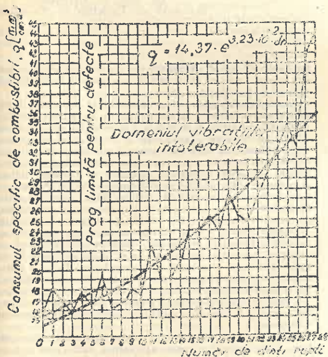
Fig. 1. Dependența dintre numărul de dinți rupți și consumul de combustibil.
