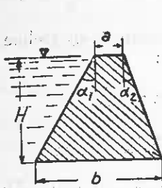
Fig. 9. Profil trapezoidal asimetric cu fruct amonte și aval.
