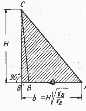
Fig. 4. Profil triunghiular economic.
