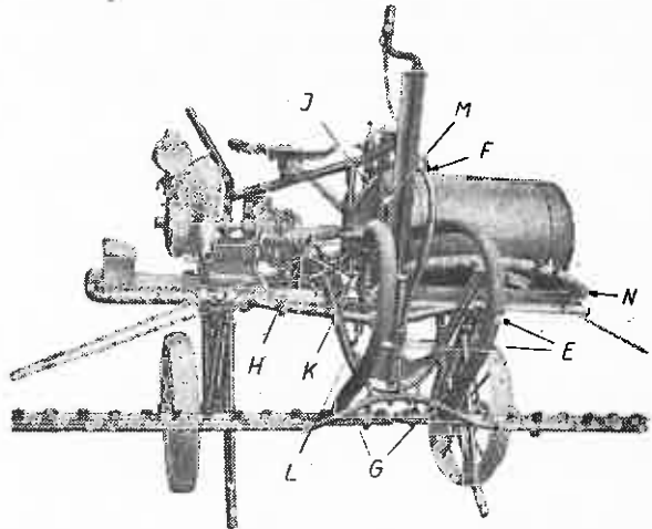
Fig. 2. Mașina combinată PSN 6 pentru stropit și prăfuit.
