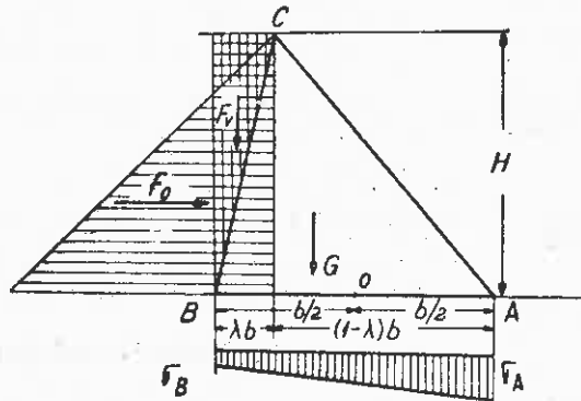
Fig. 3. Profil teoretic (triunghiular).
