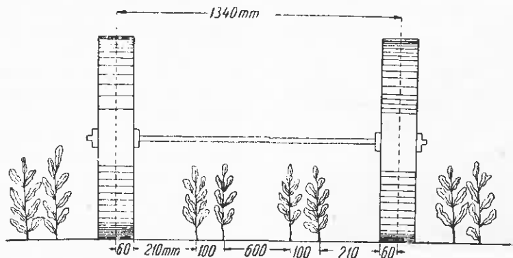
Fig. 4. Inscrierea roților mașinii de stropit OTP între rândurile de puieți (după formula ing. I. F. Snegovski).
