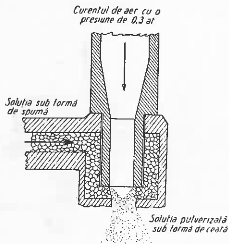
Fig. 3. Principiul de pulverizare a mașinii PSN 6.
