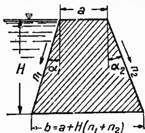
Fig. 7. Secțiune printr'un baraj cu ambele paramente înclinate.
