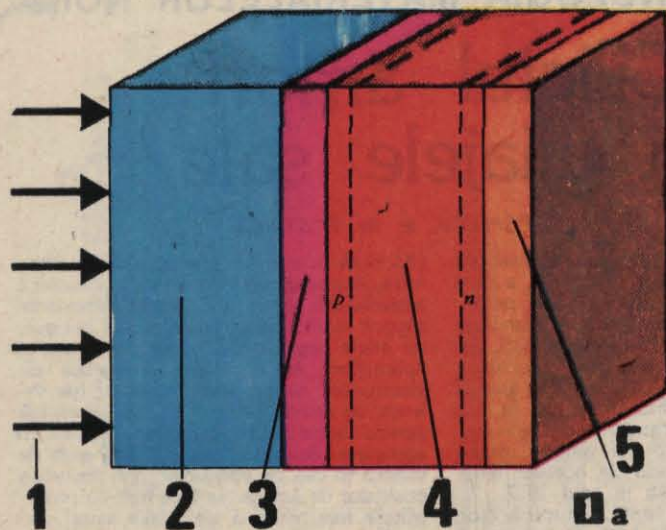
Fig. 1. a) Structura celulei p-n cu a-Si:H; b) celule integrate cu a-Si:H. 1 — lumină; 2 — sticlă; 3 — electrod transparent; 4 — a-Si:H; 5 — electrod metallic.
